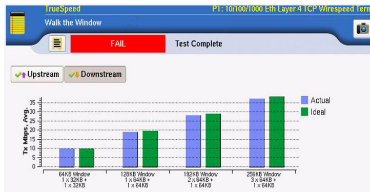
그림 7. Walk-the-Window 테스트 화면 - 다운스트림
