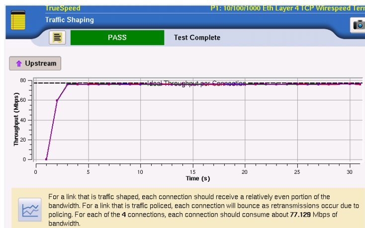
그림 18. TrueSpeed Traffic Shaping 결과(트래픽이 정형화되는 경우)
