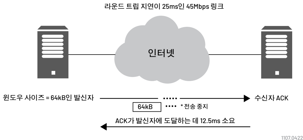
그림 1. RTD가 25ms인 45Mbps WAN 링크에서의 TCP 처리 중 데이터 바이트 그림
