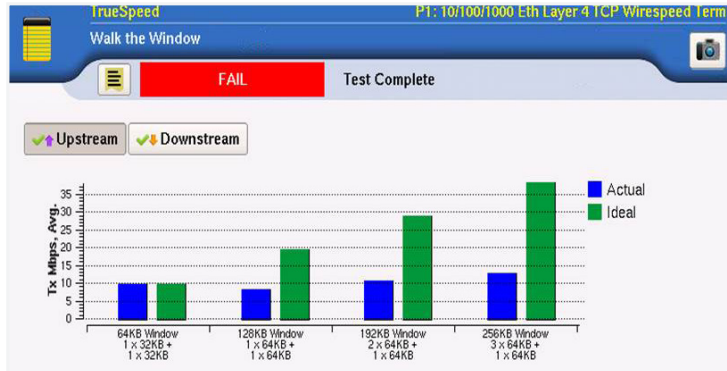
그림 6. Walk-the-Window 테스트 화면 - 업스트림
