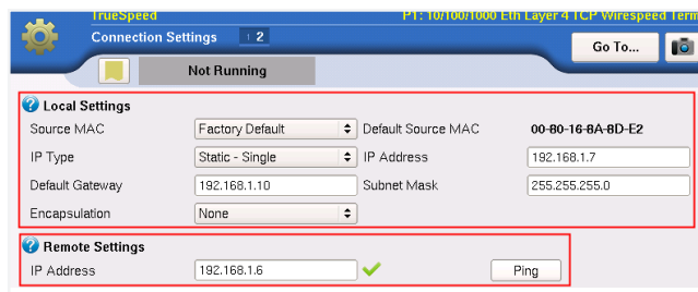
그림 3. IP 주소 구성
